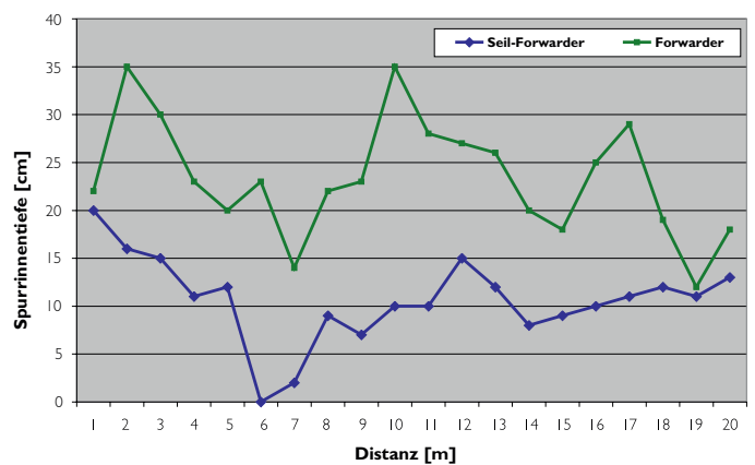
BOKU-Studie belegt halbe Einsinktiefe bei Seilforwarder. Wratschko 2006.
